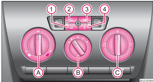
Obr. 122 Climatic: ovládací prvky
