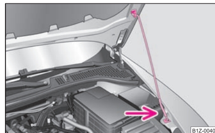
Obr. 196 Zajištění vika motorového prostoru vzpěrou
