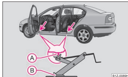
Obr. 215 Výměna kola: body pro nasazení zvedáku
