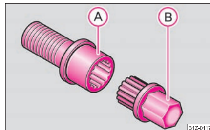
Obr. 216 Bezpečnostní šroub s adaptérem
