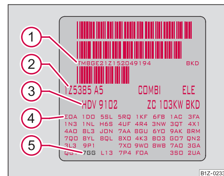
Obr. 239 Datový štítek
